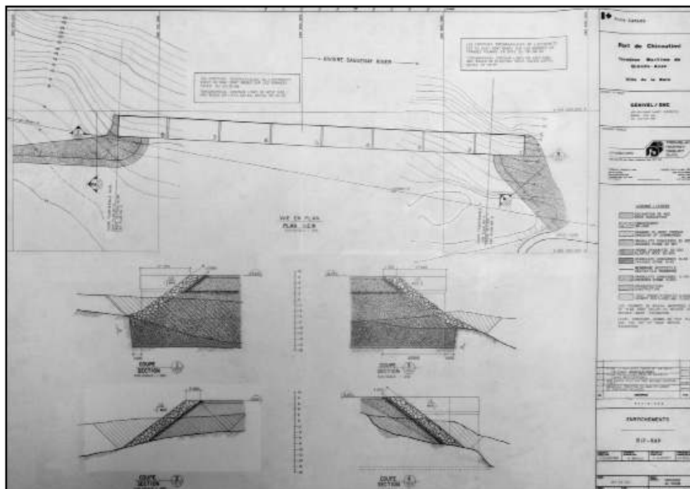
Enrochements, vue en plan. Port de Chicoutimi, Terminus Maritime de Grande-Anse, Ville de la Baie. Date : 84-02-03 SHS-F0085,1398,planche 13
